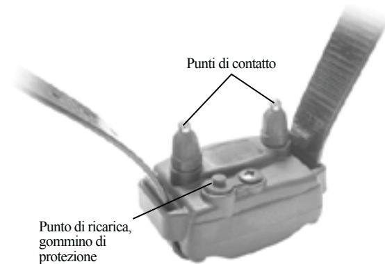
Collare Ricevitore
