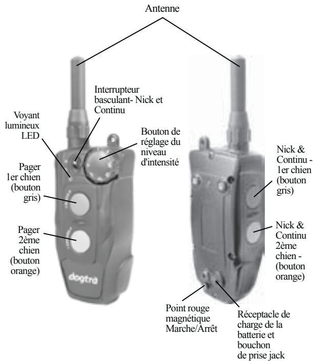
612C Emetteur
