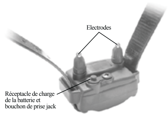
Récepteur
